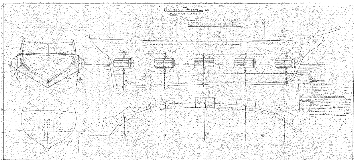
Γενική Διάταξη του Πάρων «Άρης». Η εικόνα παραχωρήθηκε από το Ναυτικό Μουσείο της Ελλάδας.
